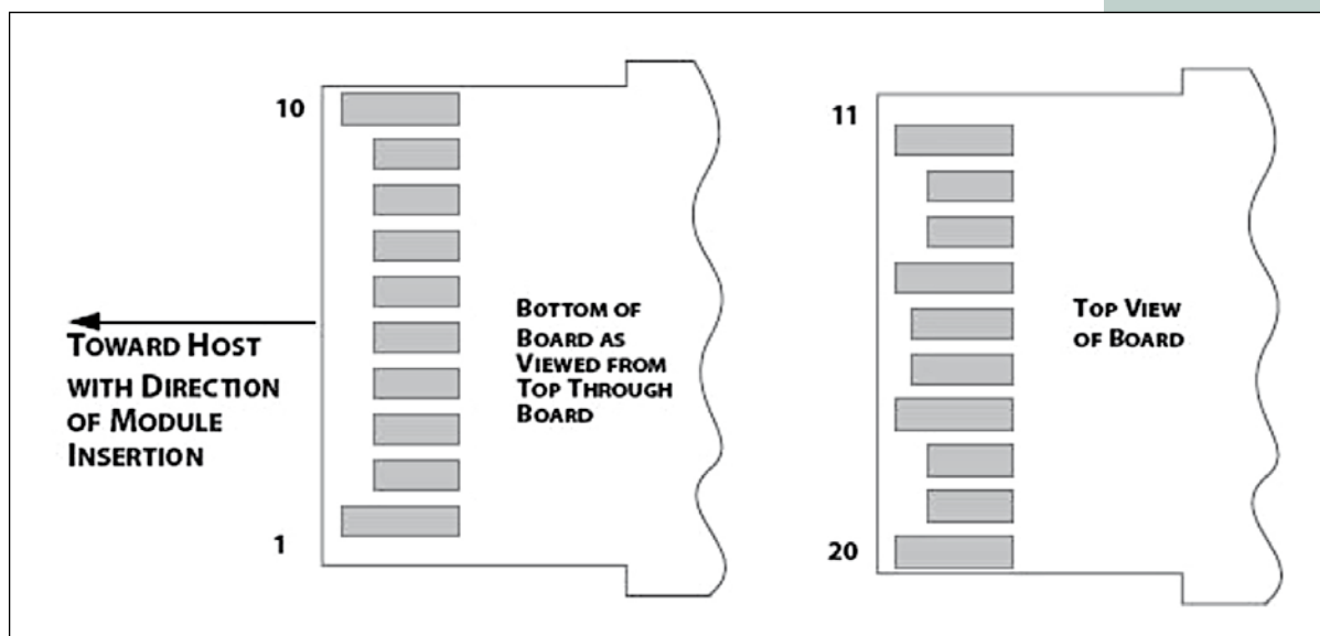
Figura 3: Asignación de contacto del módulo
