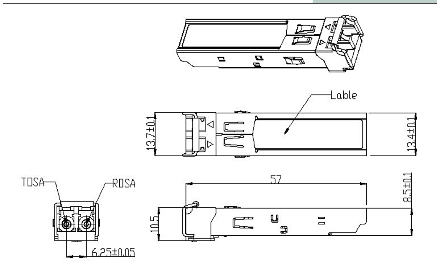
Dimensiones mecánicas
